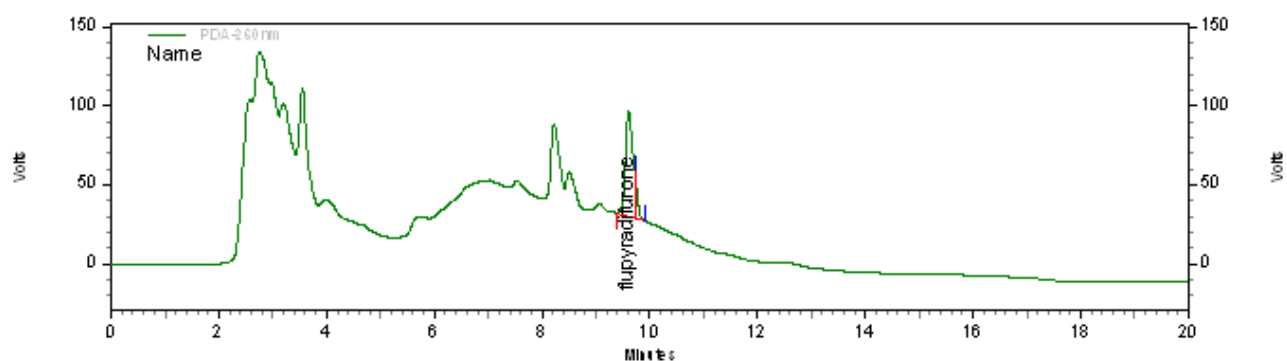
Рис. 7. Хроматограмма экстракта из почвы, содержащей флупирадифурон в максимальной тестируемой концентрации 5 мг/кг.
