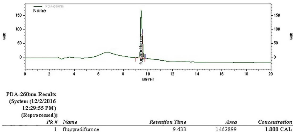
Рис. 4. Хроматограмма водного стандарта флупирадифурона в максимальной ( 1 \text{ мкг/см}^3 ) концентрации из градуировочного графика.
