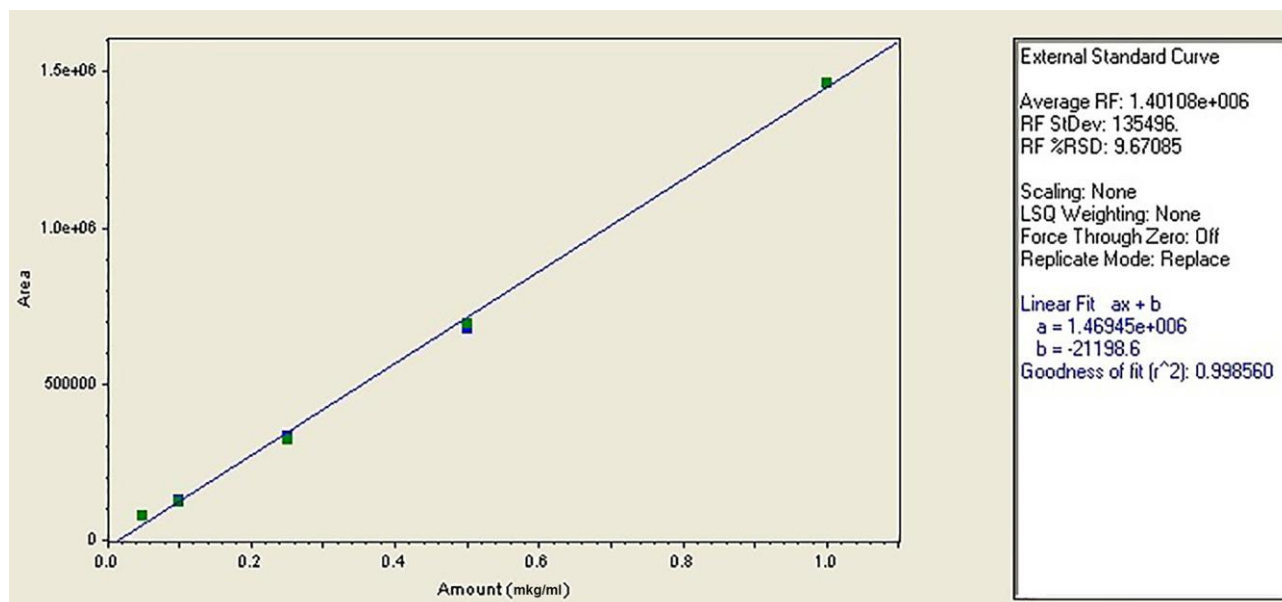
Рис. 2. Градуировочный график, отражающий зависимость среднего значения площади пика на хроматограммах от концентрации флупирадифурона в растворе (мкг/см 3 ).
