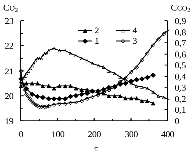
Рис. 4. Изменение концентрации диоксида углерода ( C_{\text{CO}_2} ) и кислорода ( C_{\text{O}_2} ) в реакторе: при 20^\circ\text{C} : ◇ - \text{CO}_2 (3); Δ - \text{O}_2 (4); при 5^\circ\text{C} : ◆ - \text{CO}_2 (1); ▲ - \text{O}_2 (2). C_{\text{CO}_2} - концентрация \text{CO}_2 (% об.); C_{\text{O}_2} - концентрация \text{O}_2 (% об.); \tau - время (мин).
